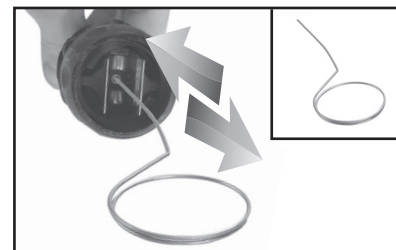
Ihla na čistenie trysky, Obr.13
