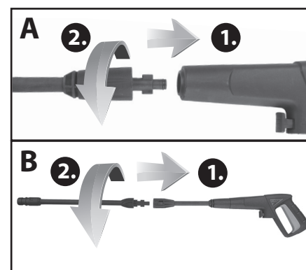
Nasazení nástavců na stříkácí pistoli čističe 43103 Obr.4
