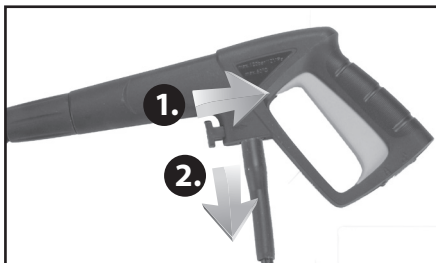
A magasnyomású tömlő leválasztása a pisztolyról, 7. ábra
