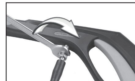
Montáž tlakovej hadice k pištoľi u modelu HPC 1800 Obr.8
